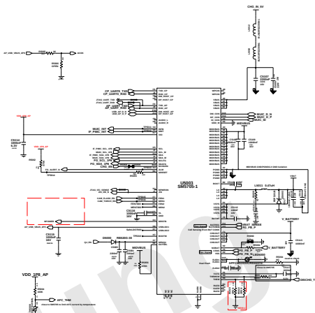
IF PMIC (SM5705)
